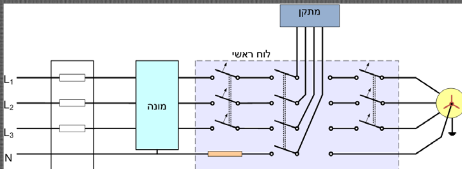
מפסק מחלף 4 קטבי לוח ראשי של המתקן
