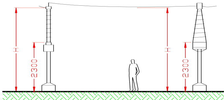
איור 12: התקנת צידוד מ"ג – ללא מחיצות מגן
