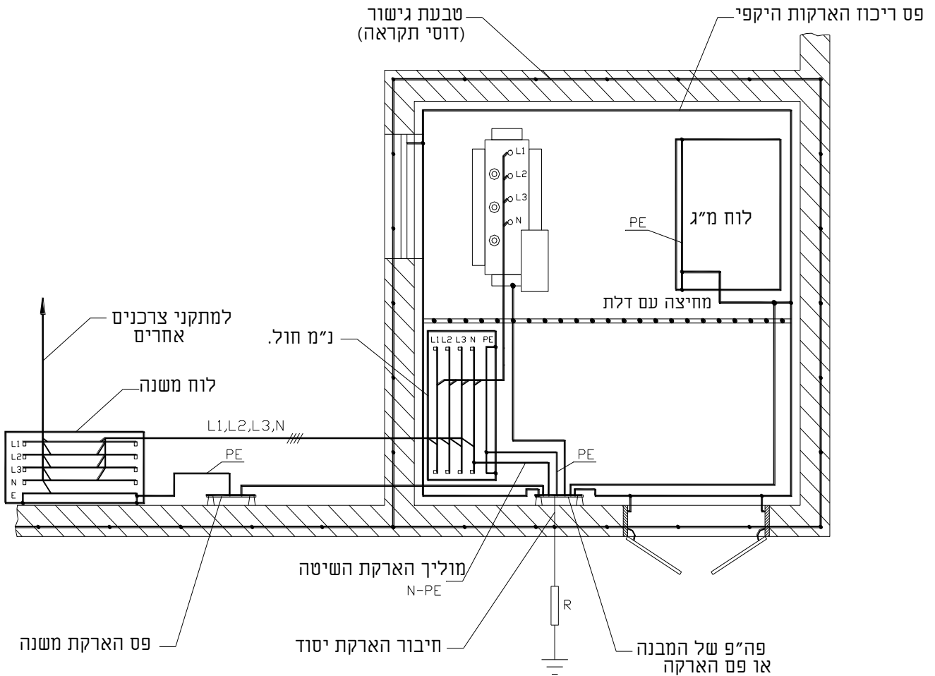
איור מס' 21 דוגמת תחט"פ המזינה לוח ראשי ולוח משנה במבנה אחד – ביצוע הארקה המשותפת
