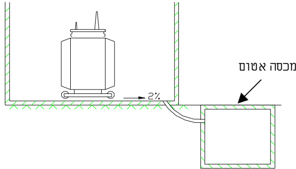
איור 5: התקנת שנאי על רצפה רגילה עם בור איסוף חיצוני
